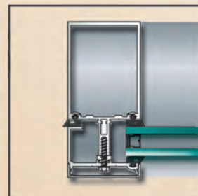
JAMBS
